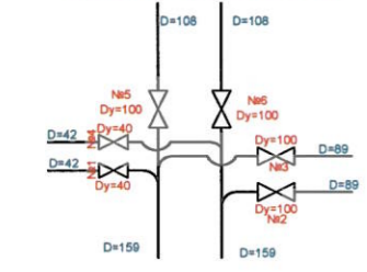
Тепловая камера № 1 в Торфяники (2-х этажные)
