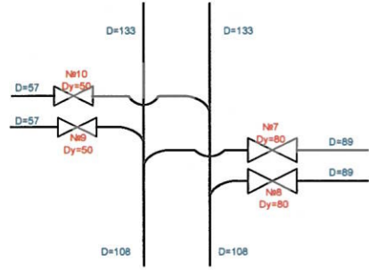
Тепловая камера № 2 в Торфяники (2-х этажные)
